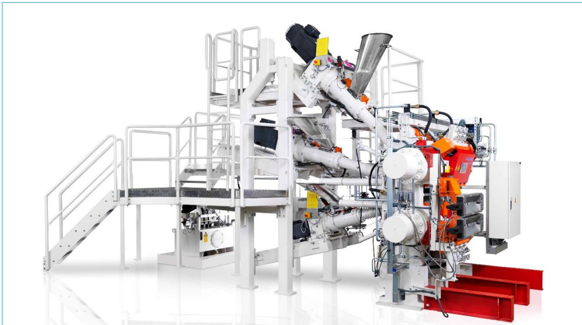
Multiplex-Extrusionsanlage zur Herstellung von Reifenlaufstreifen [Bild: KraussMaffei Extrusion GmbH]
