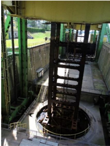
Hebetechnik für den Trog
